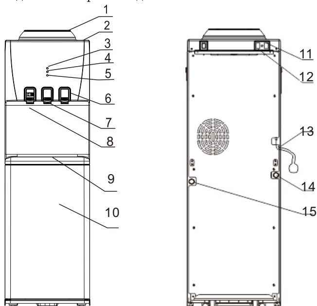
Рис.1. Схема аппарата CH-V130
