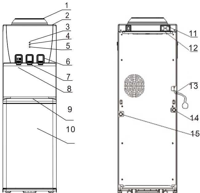
Мал. 1. Схема апарату CH-V130
